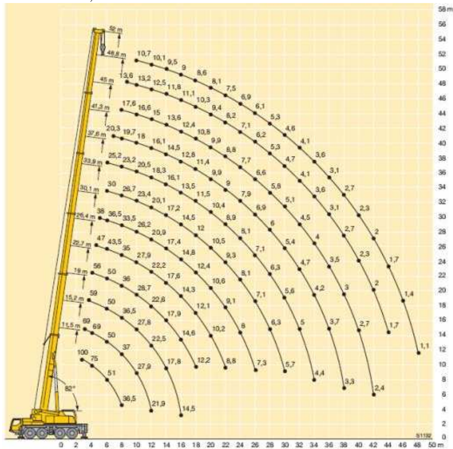
Jeřáb 110 tun, radius 13 tun max. 18m
