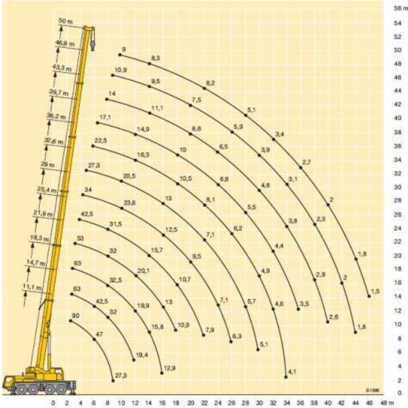
Jeřáb 110 tun, radius 13 tun max. 18m
